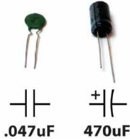
चित्र 1.2.1 (एफ) कैपेसिटर
