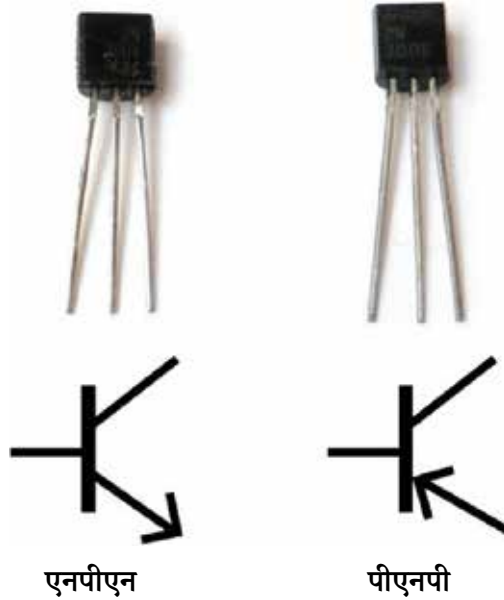
चित्र 1.2.1 (एच) ट्रांजिस्टर
